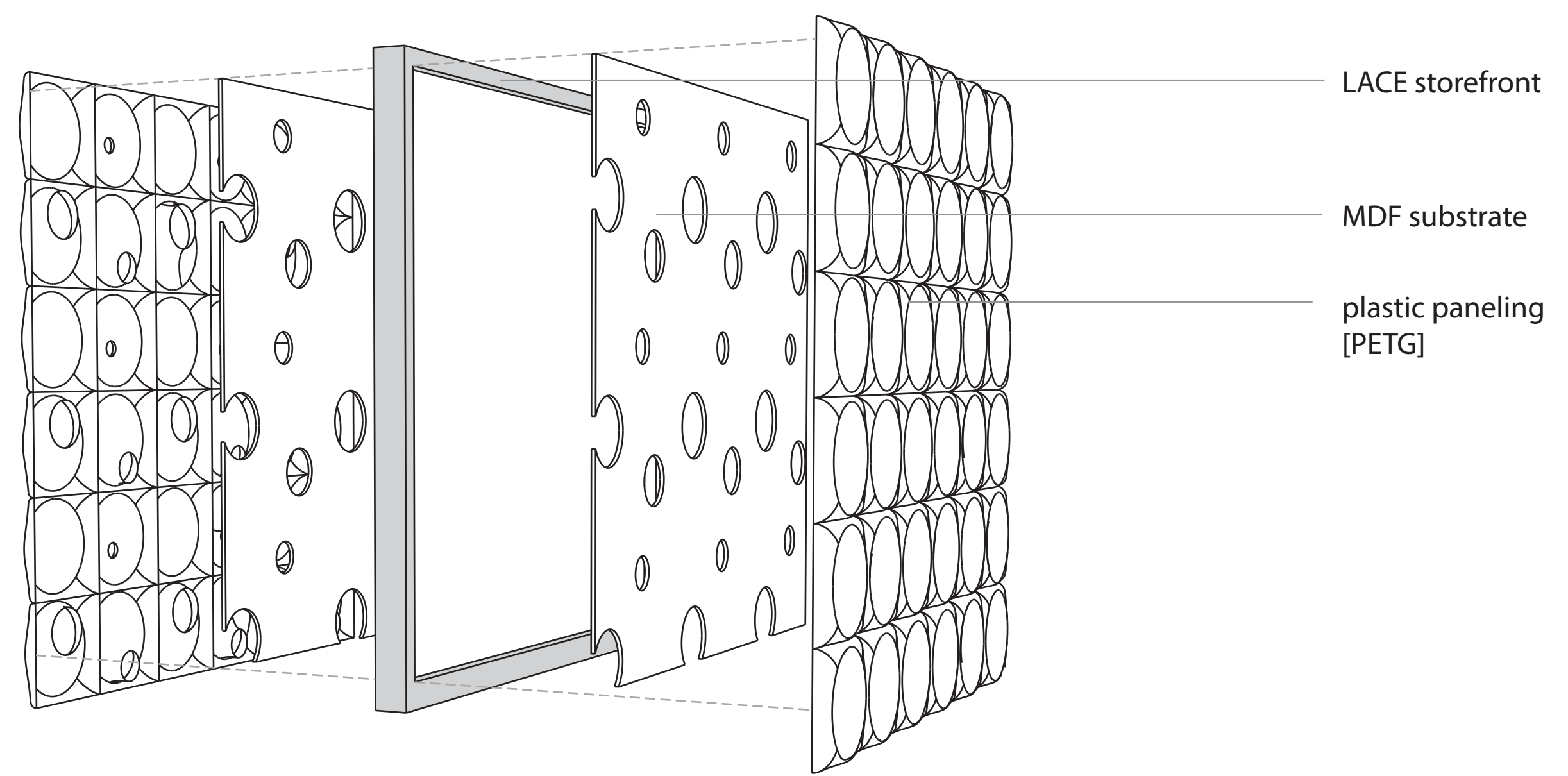
ASSEMBLY AXONOMETRIC
